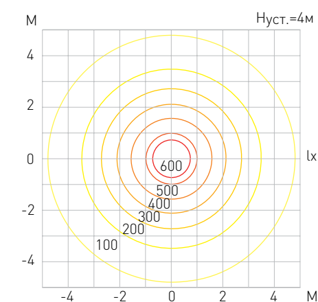
Диаграмма освещенности для TAİKO 1500 LED 3000K
